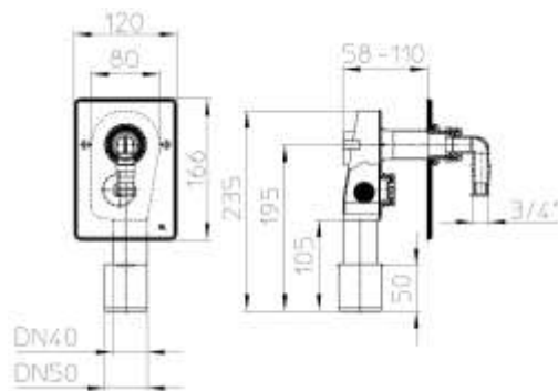
Рис. 1. Встроенный сифон HL400.
